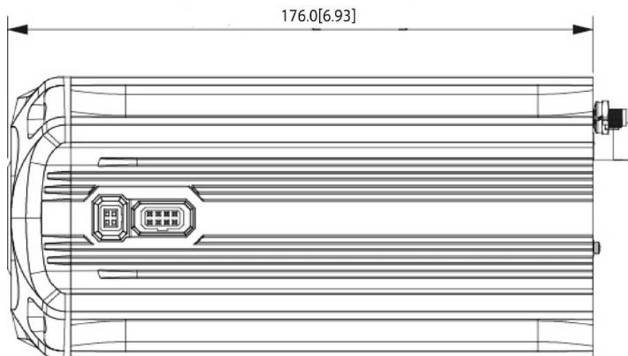
图2-5 侧面板尺寸图 (单位: mm[inch])
