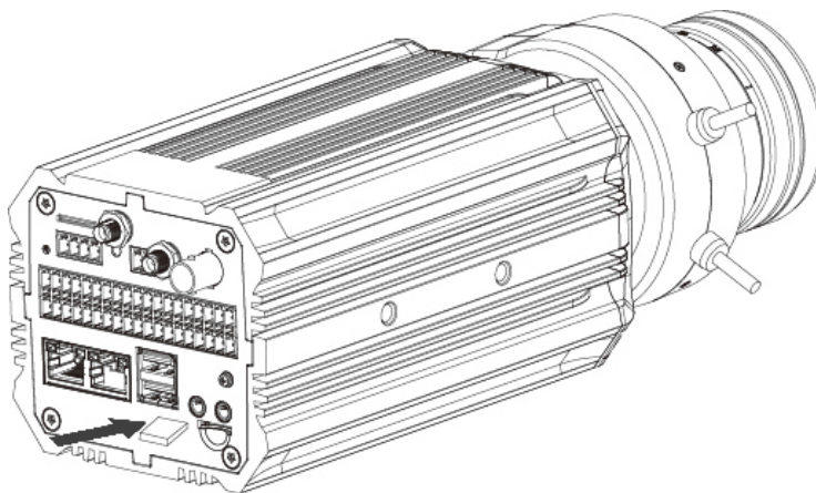
图3-3 安装 TF 卡
