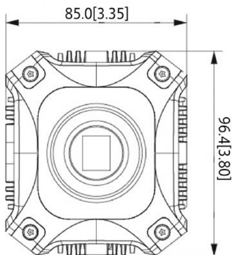
图2-6 前面板尺寸图（单位：mm[inch]）
